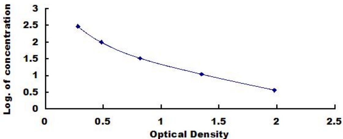
牛磺胆酸(TCA)检测试剂盒标准曲线
