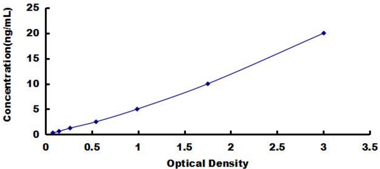
人血管生成素样蛋白 2 (ANGPTL2) 检测试剂盒标准曲线
